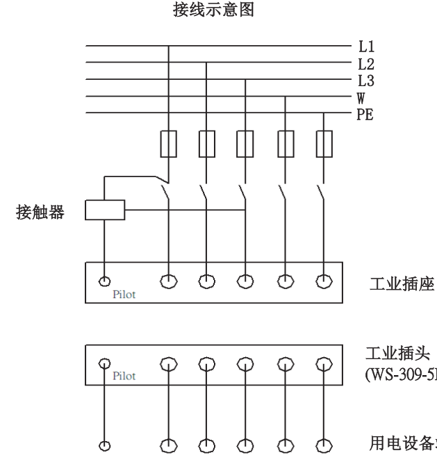
图示4 接线示意图
