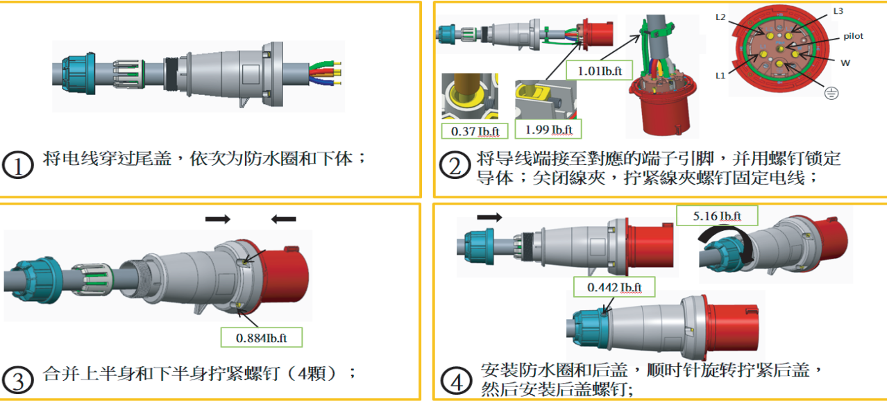
圖示2 接線組裝流程图
