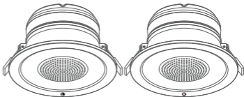
智能可調光藍牙音樂LED嵌燈 -雙聲道
