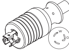
WS-118-5 NEMA L5-15P
