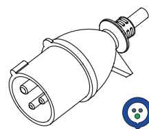
WS-197-1-P2 2P3W-16A-6H 200-250V~
