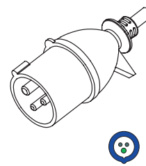
WS-197-1 2P3W-16A-6H 200-250V~
