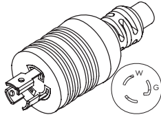
WS-118 NEMA L5-15P
