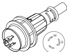
WS-118-2 NEMA L5-15P
