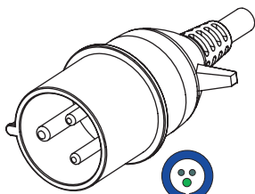
WS-309-3P-32A-6H-P-1 2P3W-32A-6H 200-250V~
