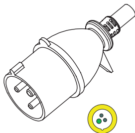
WS-196-1 2P3W-32A-4H 100-130V~
