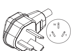
WS-001J-1 NEMA 10-50P
