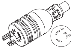
WS-226 NEMA L7-15P
