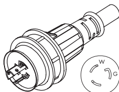
WS-226-2 NEMA L7-15P
