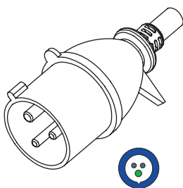
WS-196 2P3W-32A-6H 200-250V~
