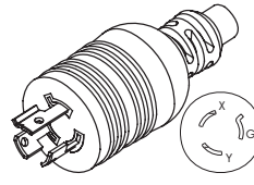
WS-123 NEMA L6-15P
