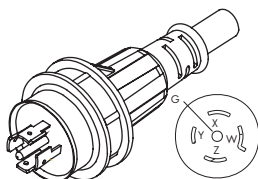
WS-234-2 NEMA L21-20P
