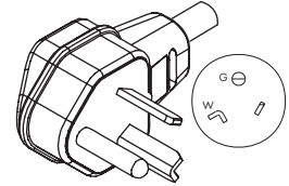
WS-001R NEMA 7-30P
