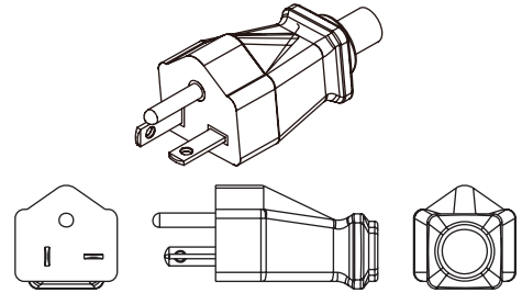
WS-001I-6 Cable "L"
