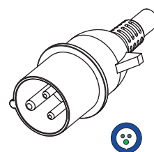
WS-309-3P-16A-6H-P-1 2P3W-16A-6H 200-250V~
