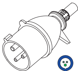
WS-196-P2 2P3W-32A-6H 200-250V~
