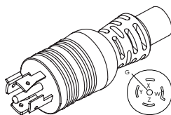
WS-223 NEMA L22-20P
