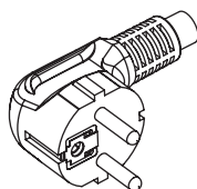
WS-010E (15A 250V)
